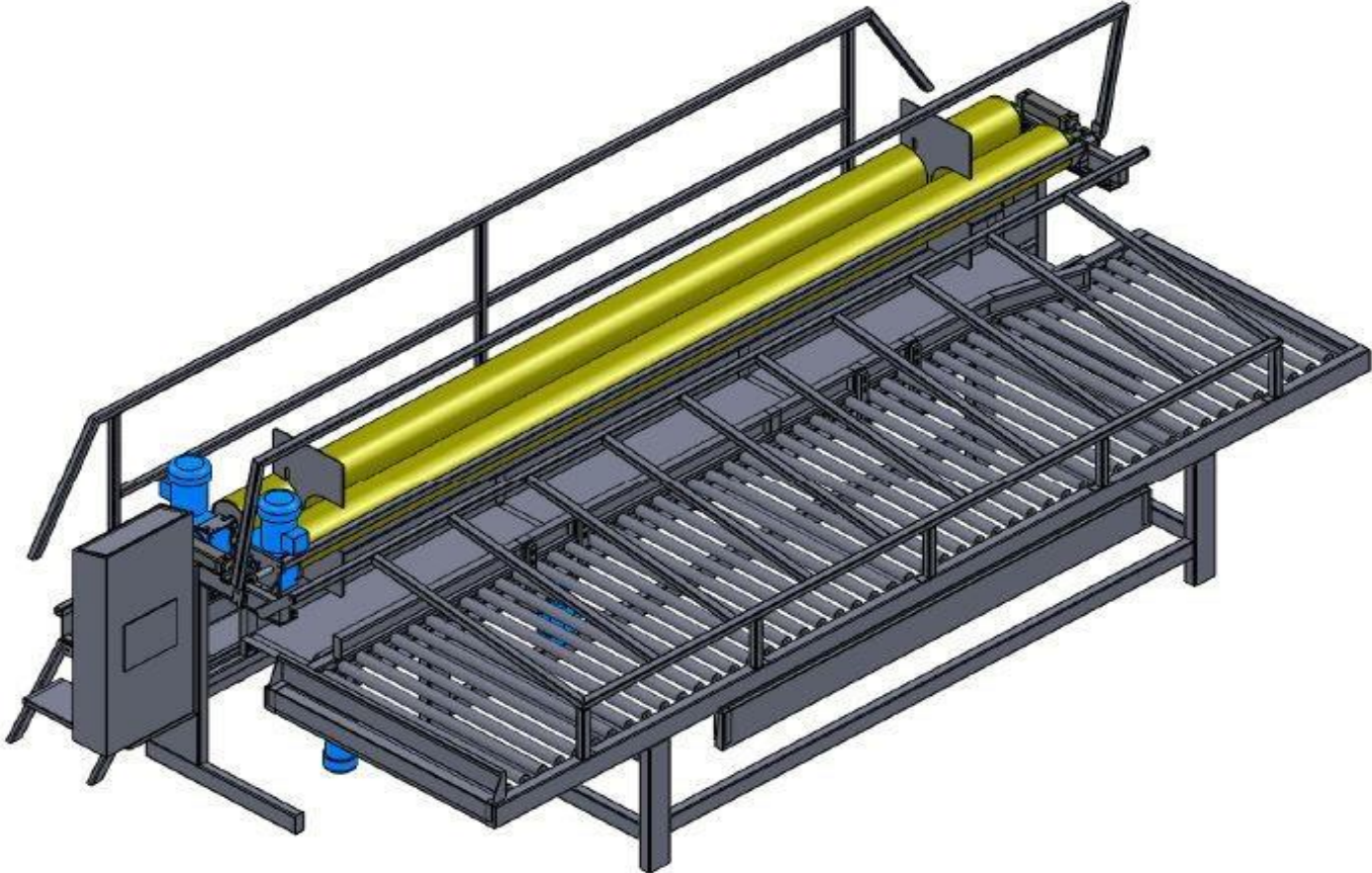
- Semi Automatic Winding Machine / Yarı Otomatik Halı Sarım Makinesi
