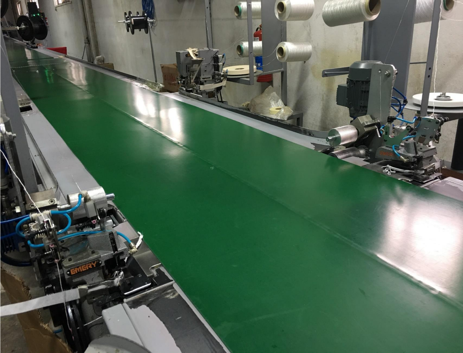
- Short Side Right-Left Overedge Line / Kısa Kenar Dikiş Sürfile Hattı
